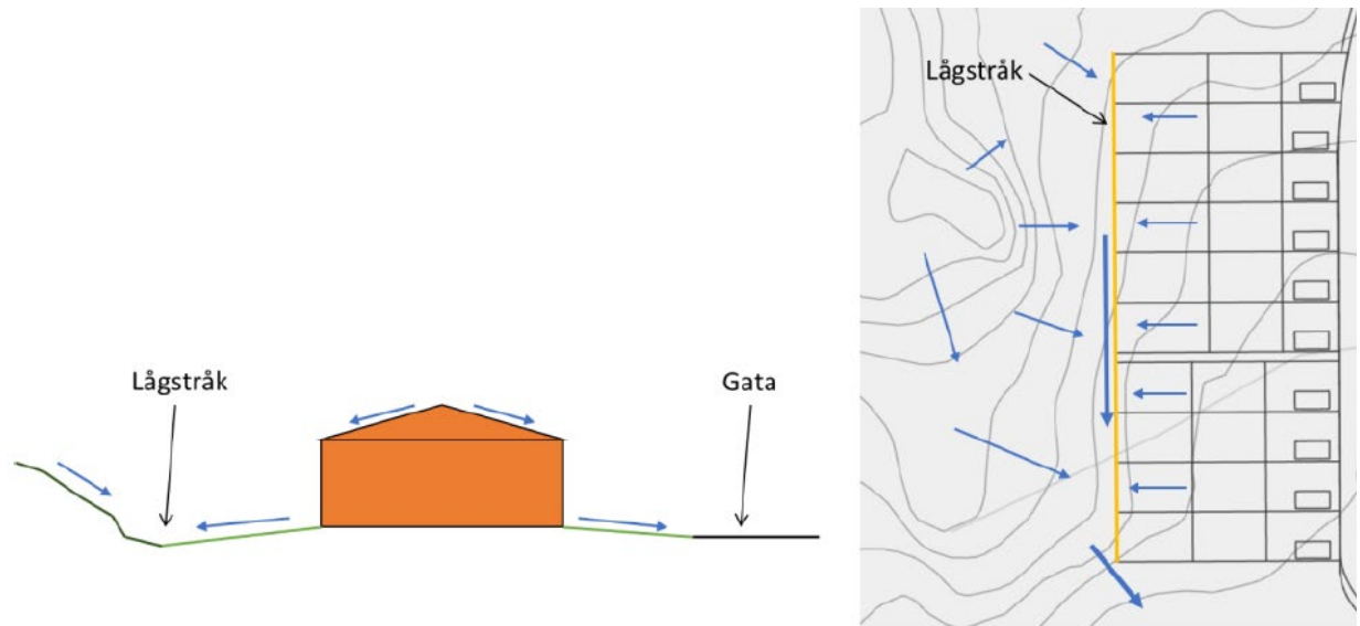
Figuren ovan till vänster visar princip för placering av hus, höjdsättning av kringliggande mark samt tillskapande av sekundära flödesvägar för att hantera skyfall. Figuren till höger visar hur principen kan appliceras på ett delområde om exploatering sker med radhus (WSP Samhällsbyggnad).
