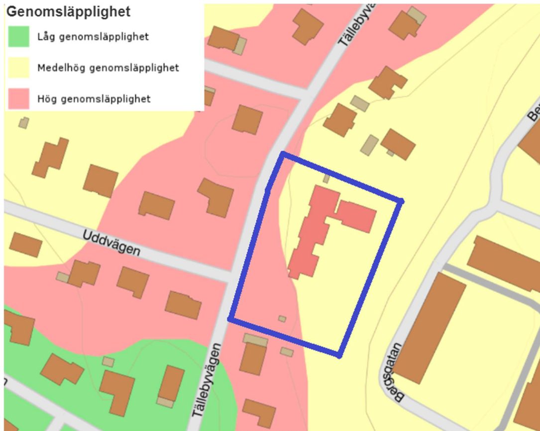
Figur 5. Genomsläpplighet/Infiltrationskapacitet (SGU)
