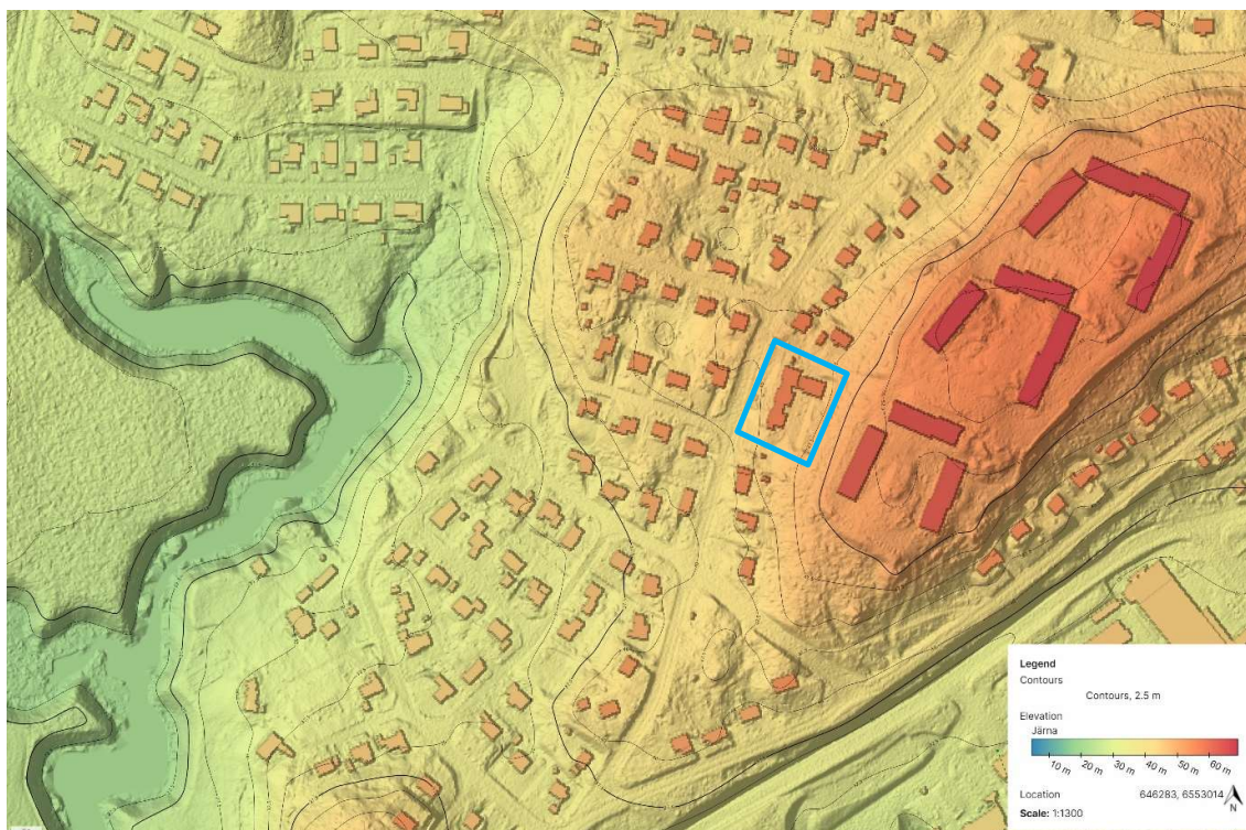
Figur 3. Topografi
