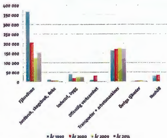
CO 2 -utsläpp i Södertälje 1990-2014 (ton/år) Fjärrvärmens är den sektor där utsläppen av koldioxid har minskat mest. Utsläppen från transporter ligger högst 2009 och har successivt ökat sedan 1990.
