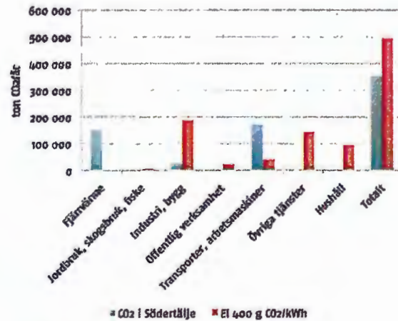
Direkta CO 2 -utsläpp i Södertälje och CO 2 -utsläpp från el 400g/kWh (ton/år)
