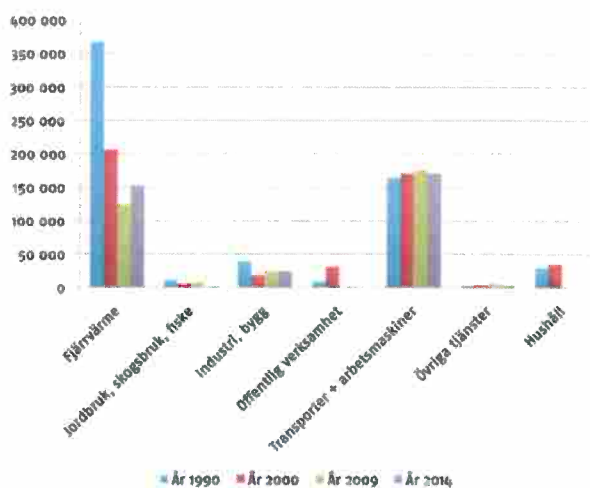
CO2-utsläpp i Södertälje 1990-2014 (ton/år) Fjärrvärmens är den sektor där utsläppen av koldioxid har minskat mest. Utsläppen från transportererna ligger högst 2009 och har successivt ökat sedan 1990.
