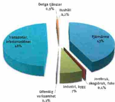
CO2-utsläppen i Södertälje 2014 (procent) Transporter bidrar med de största utsläppen av koldioxid och därefter fjärrvärmeproduktionen. Industri och bygg kommer därefter. Övriga tjänster är handel, kontor, hotell med mera. Hushållens andel är den eldningsolja som finns kvar för uppvärmning av bostäder.
